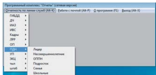
Рис.2. Клиентская программа
