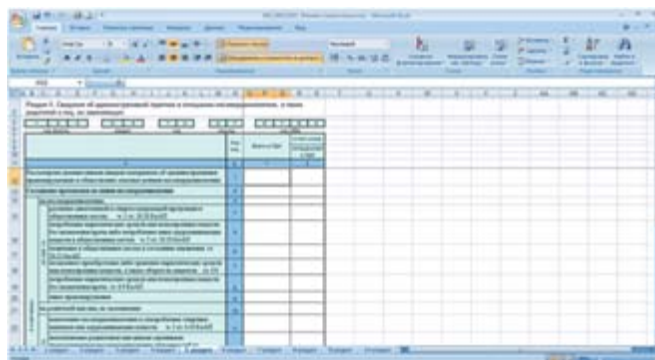
Рис.4. Форма отчетности
